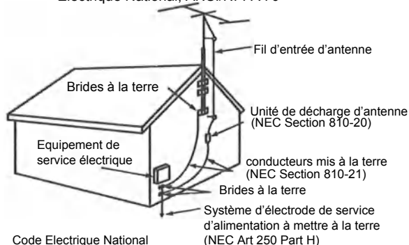
Mise à la terre d'antenne selon le Code Electrique National, ANSI/NFPA 70
