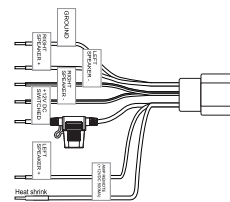
Faisceau de câblage
