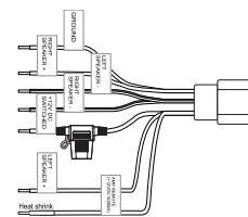
Árnés de cableado
