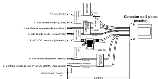
Vista B-B Vista de inserção de fios
