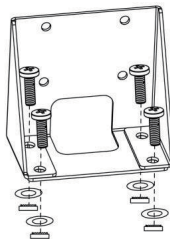
Tornillos para metales con nueces (Tamaño del agujero 7/32")
