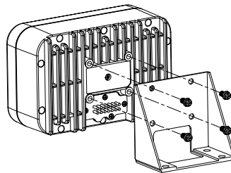
Montaje normal
