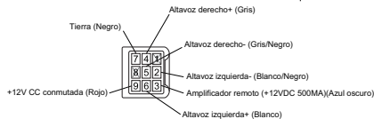
Vista B-B Vista de inserción de cables
