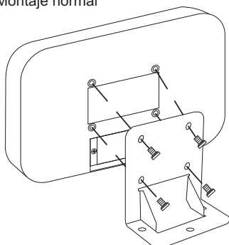
Montaje normal
