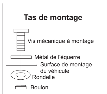
Vis mécaniques avec des boulons (Taille du trou 7/32")
